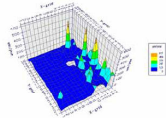
Gráfico 3D de Potencial de Media Celda.
